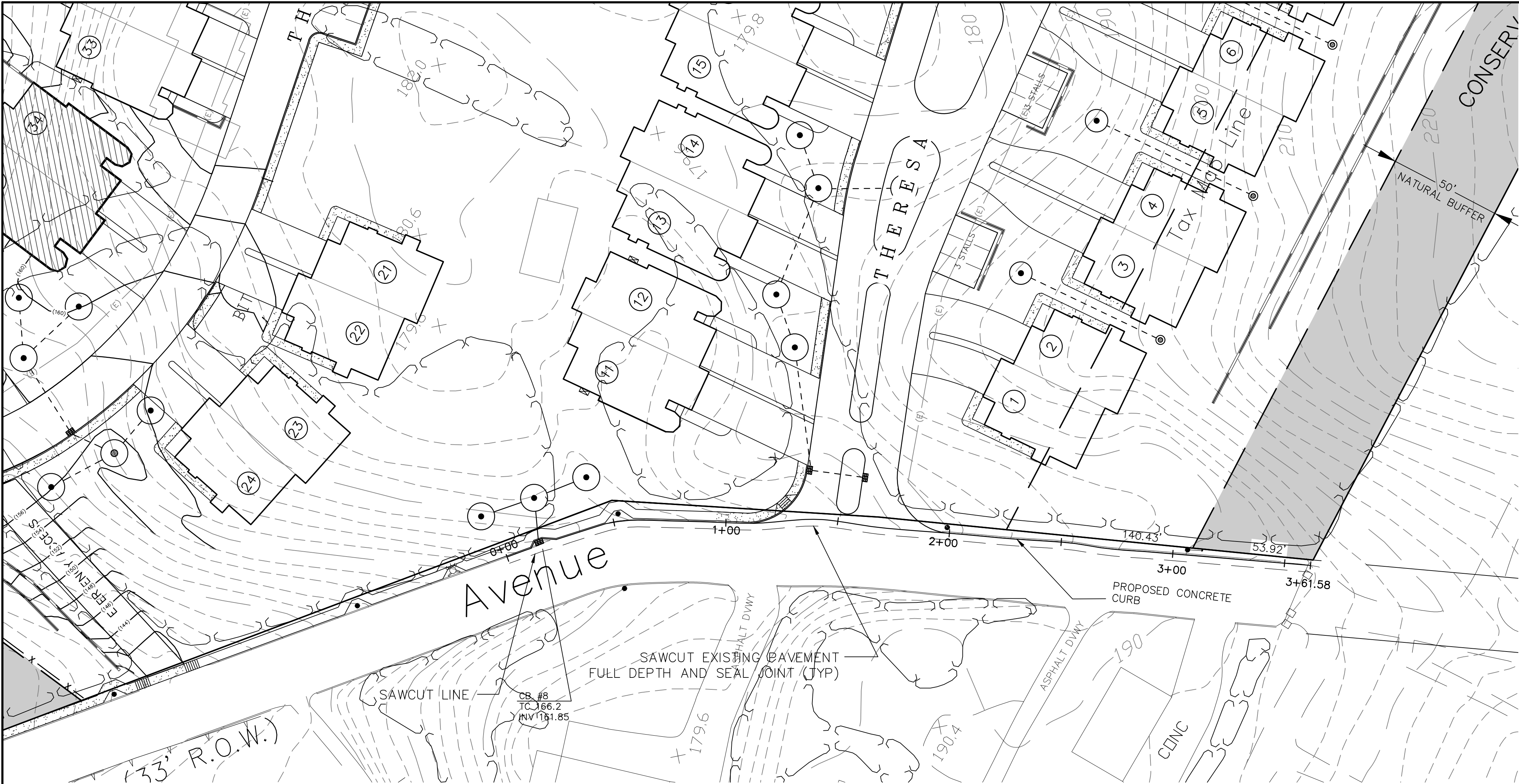
LIBERTY AVE PLAN SCALE: 1"=30'
