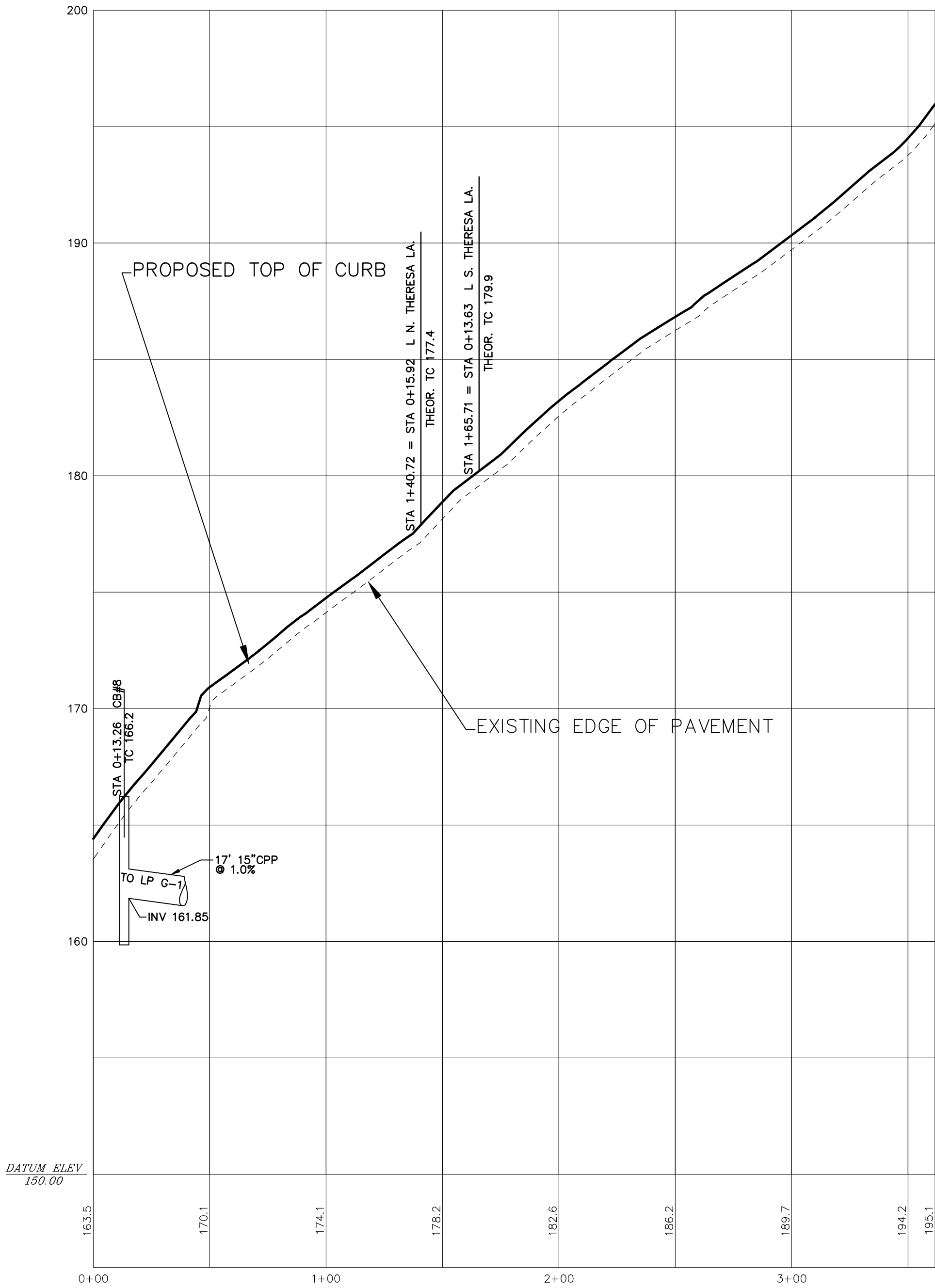
LIBERTY AVE SCALE: HORIZ. 1"=40' VERT. 1"=4'
